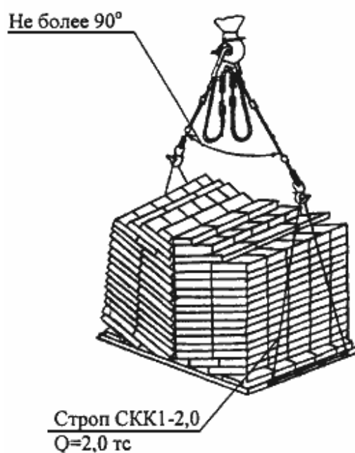
Строп СКК1-2,0 Q=2,0 тс Строп 4СК1-3,2 + 4СК1-10,0 Q = 3,2 \div 10,0 тс при разгрузке с автотранспорта кирпича на поддонах P = 1,6 т
