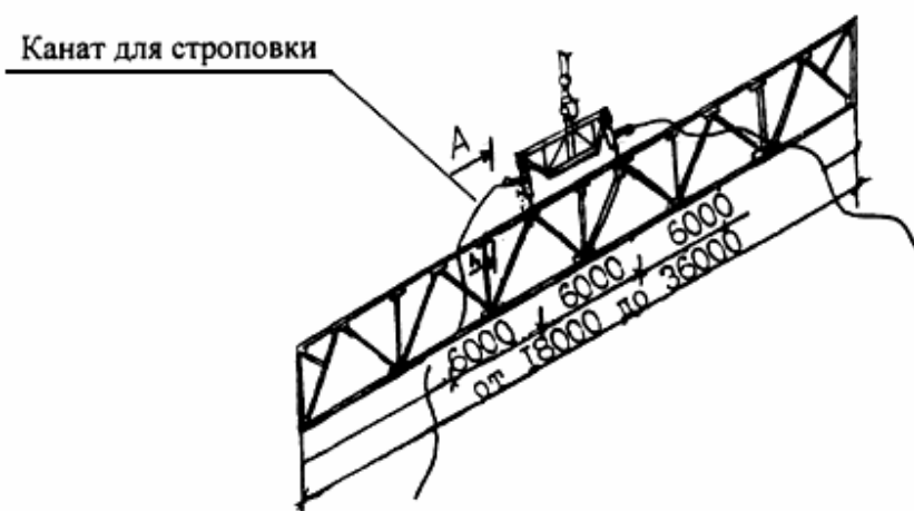
Траверса ТР 20-5,0 L = 5,42 м Q = 20 тс для монтажа металлических ферм P = 3,9 \div 15 т
