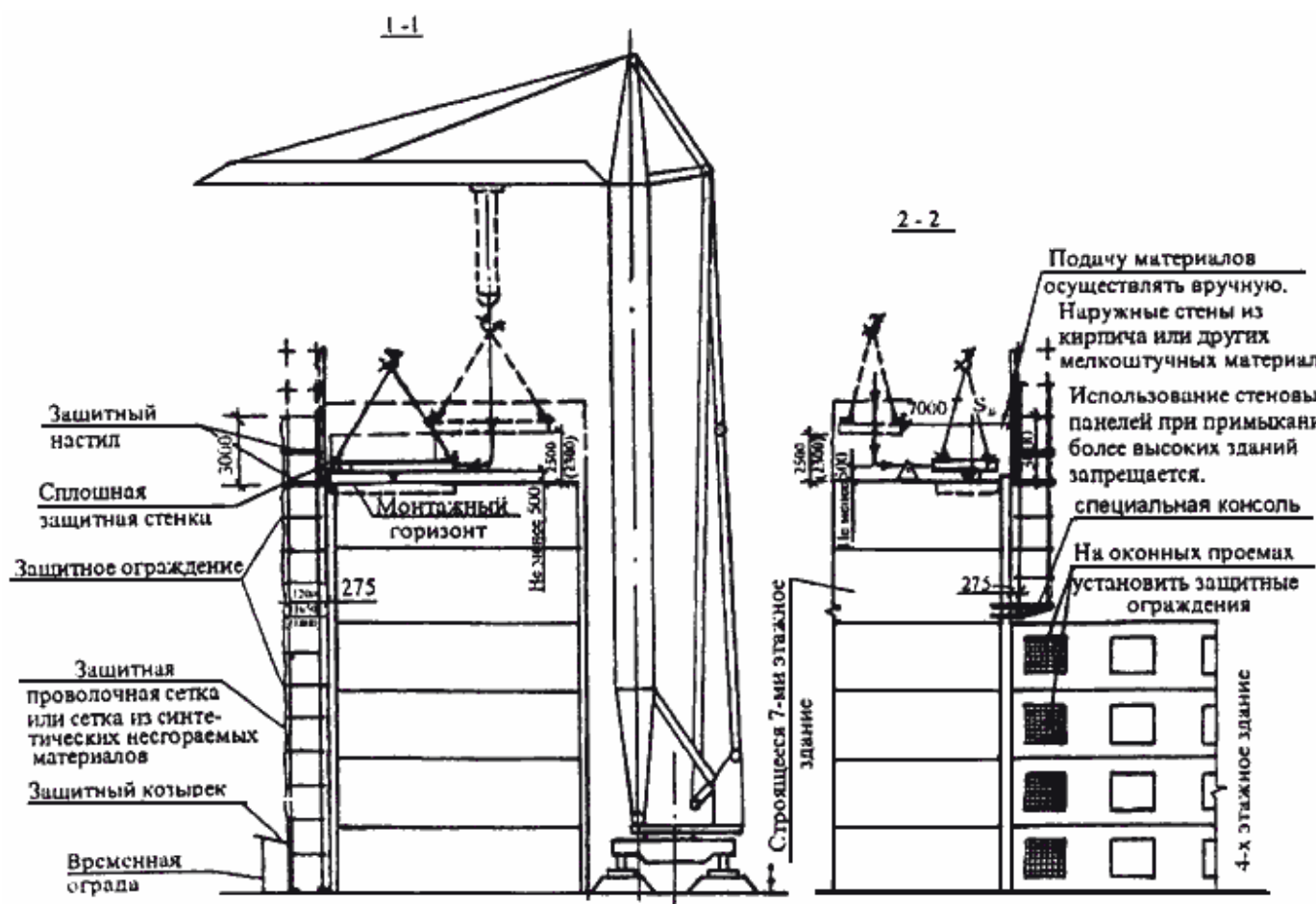
Рисунок 24 - Разрезы 1-1 и 2-2
