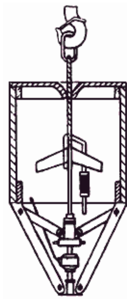
Грузозахватное приспособление для монтажа ствола мусоропровода
