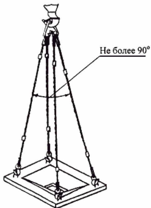
Строп 4СК1-3,2 ÷ 4СК1-10,0 Q = 3,2 ÷ 10,0 тс при монтаже капительных плит
