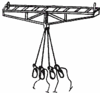
Траверса для подъема ферм покрытия двумя кранами
