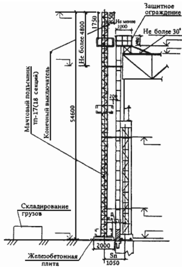
Разрез I-I
