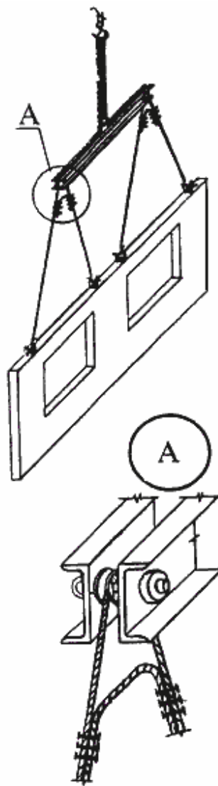
Траверса Т-1
