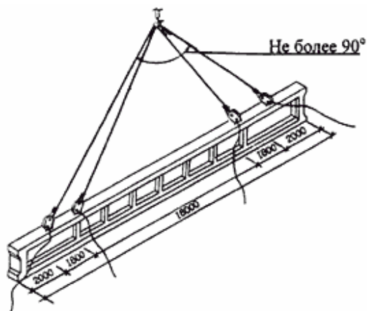
Строп 2СК-10,0
