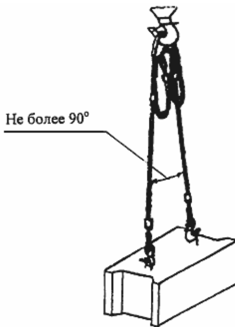
Строп 2СК-3,2 + 2СК-10,0 Q = 3,2 \div 10 тс при монтаже блоков стен подвала P = 0,31 \div 0,62 т
