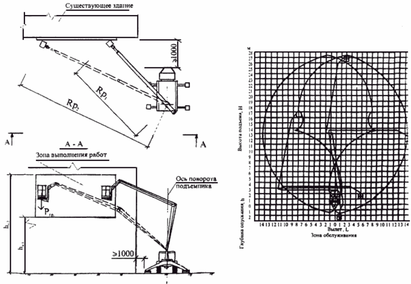
Рисунок 7 - Привязка подъемника (вышки)
