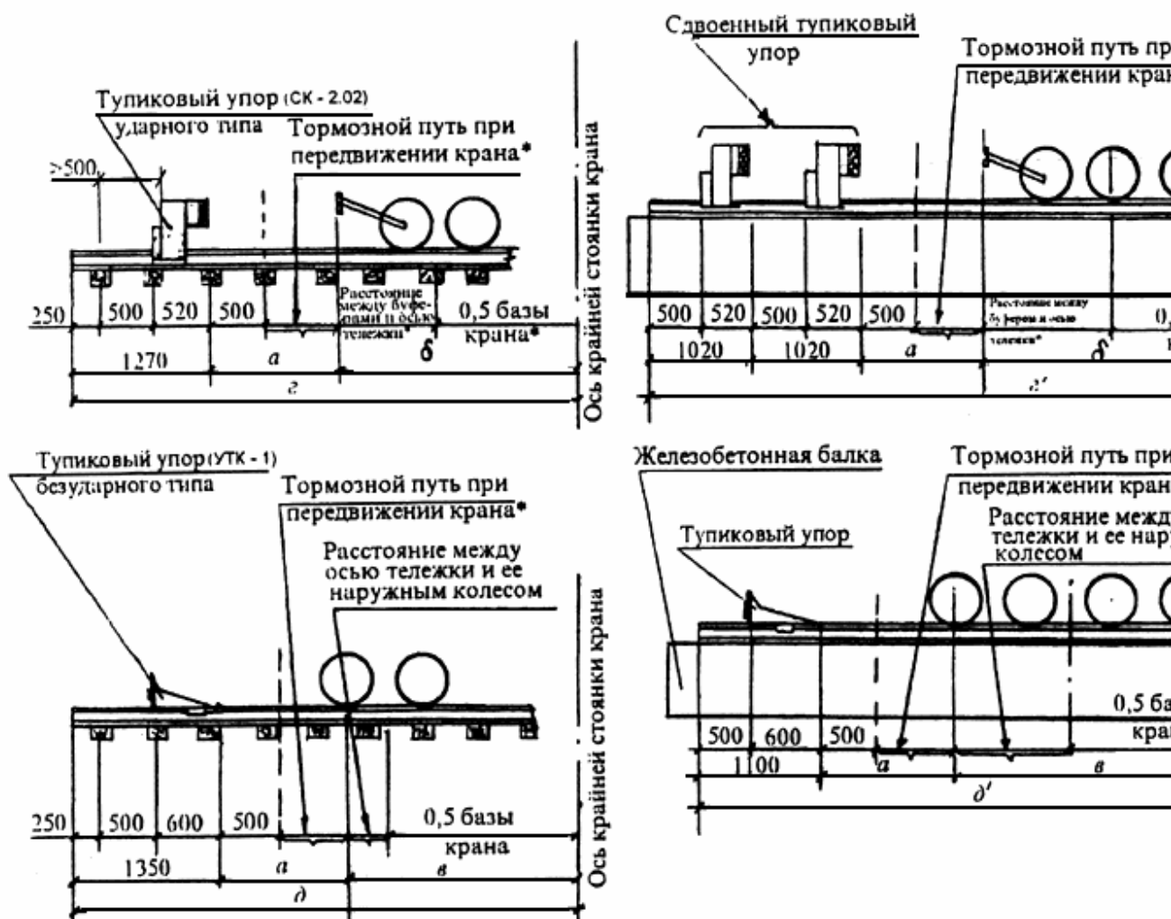
Рисунок 40 - Привязка тупиковых упоров и крайних стоянок кранов к концам рельсового пути
