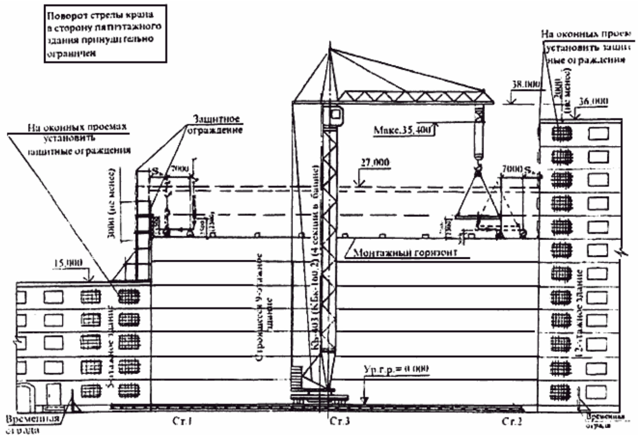
Рисунок 22 - Разрез 1-1
