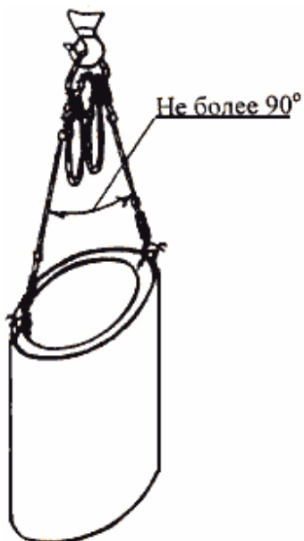
Строп 4СК1-3,2 ÷ 10,0 Q = 3,2 \div 10,0 тс при погрузке кольца горловины P = 0,06 т
