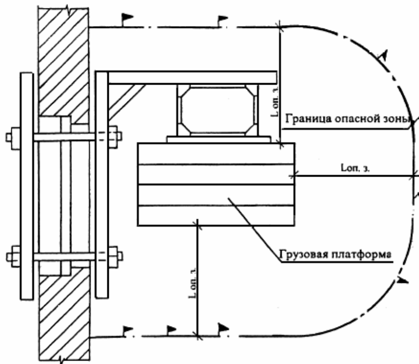
Рисунок 16 - Опасная зона при работе грузового строительного подъемника
