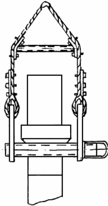
Траверса для монтажа капительных колонн
