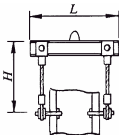
Траверса-кантователь
