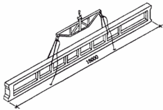
Траверса ТР20-5
