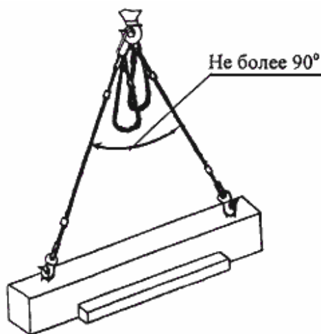
Строп 4СК1-3,2 4СК1-5,0 4СК1-10,0 Q = 3,2 \div 10,0 тс (2СК-5,0) при монтаже ригелей P = 0,3 \div 4,4 т
