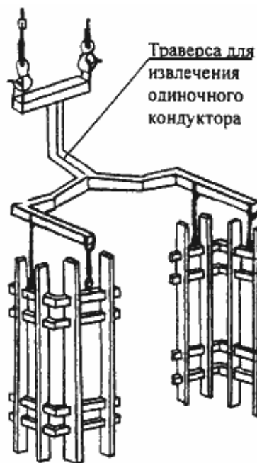
Строп 4СК1-3,2 ÷ 4СК1-10,0 при извлечении одиночного кондуктора для монтажа колонн P до 590 кг
