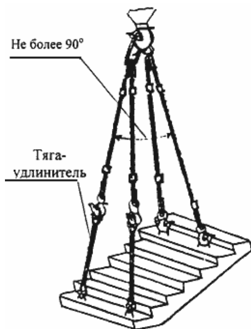
Строп 4СК1-3,2 ÷ 4СК1-10,0 Q = 3,2 \div 10,0 тс при монтаже лестничных маршей P = 0,865 \div 1,98 т
