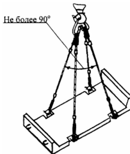
Строп 4СК1-3,2 ÷ 10,0 Q = 3,2 \div 10,0 тс при погрузке лоткового днища канала P = 0,74 \div 2,85 т
