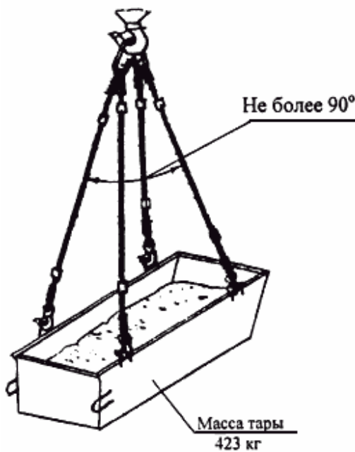
Строп 4СК1-5,0 ÷ 4СК1-10,0 Q = 5 \div 10 тс при подаче ящика с сыпучим материалом (керамзитом, гравием, песком, щебнем и т.д.) емк. 2 \text{ м}^3
