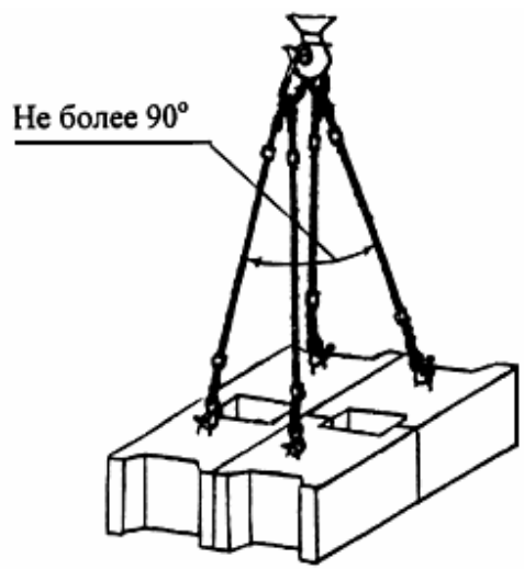
Строп 4СК1-3,2 ÷ 4СК1-10,0 Q = 3,2 \div 10 тс при разгрузке блоков стен подвала
