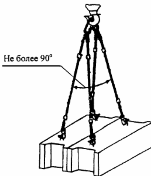
Строп 4СК1-5,0 ÷ 4СК1-10,0 Q = 5 \div 10 тс при разгрузке блоков стен подвала P = 1,96 \div 3,94 т
