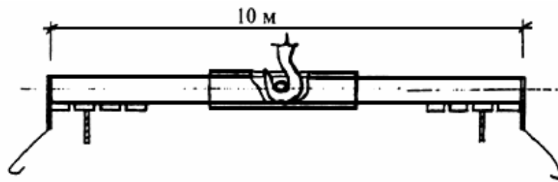
Траверса для разгрузки труб
