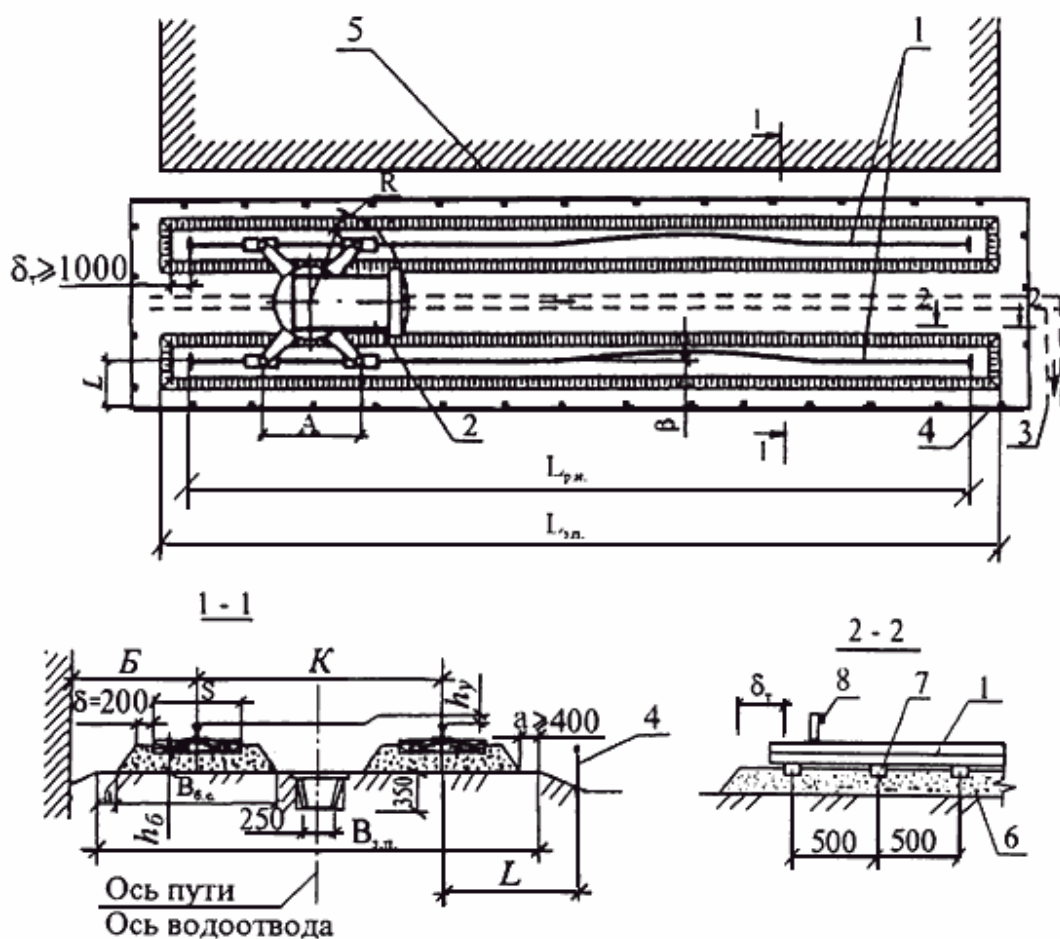
1 - рельсовый крановый путь; 2 - башенный кран; 3 - водоотводное устройство; 4 - ограждение; 5 - возводимое здание; 6 - балластная призма; 7 - полушпалы; 8 - упор тупиковый
