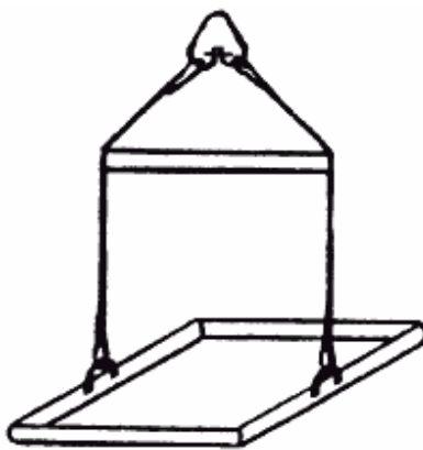
Траверса для подъема железобетонных колонн сплошного сечения
