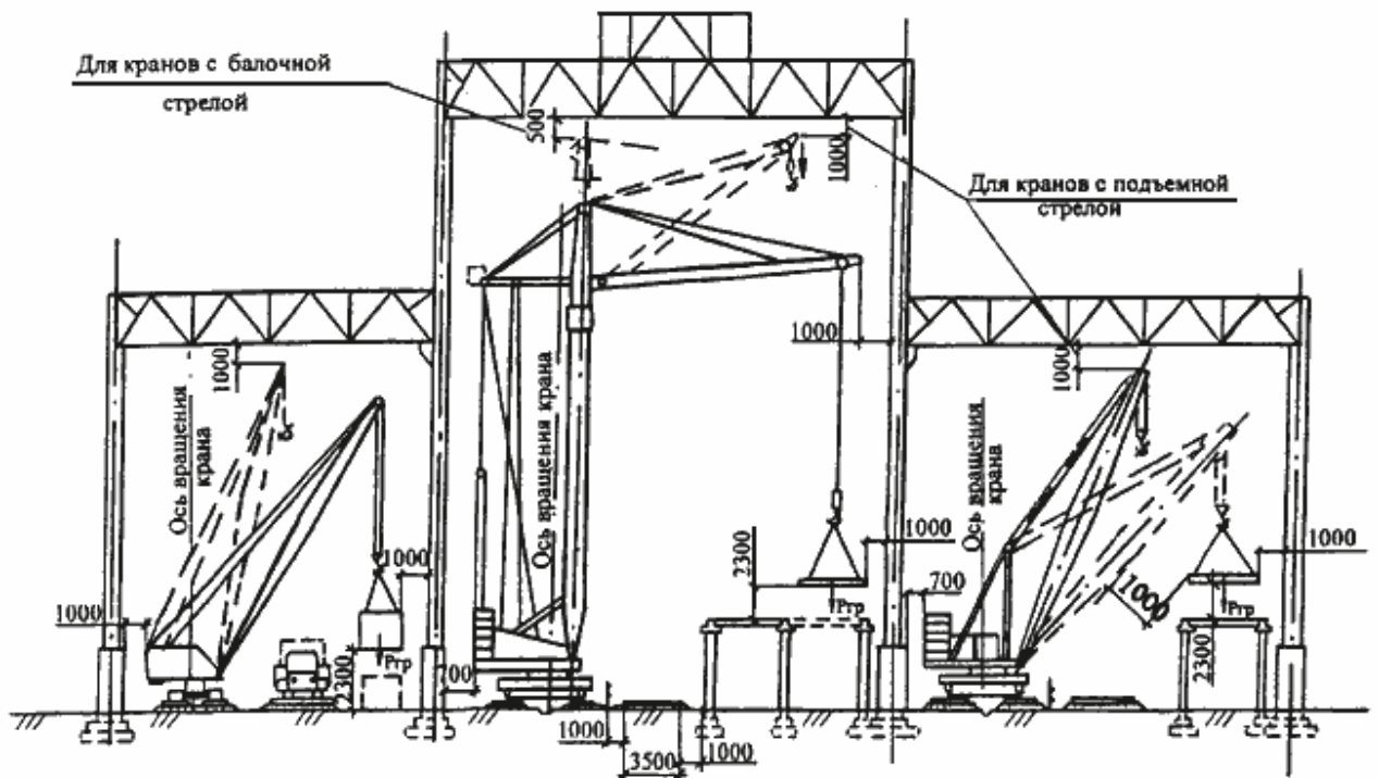
Рисунок 11 - Привязка крана внутри строящегося или реконструируемого здания
