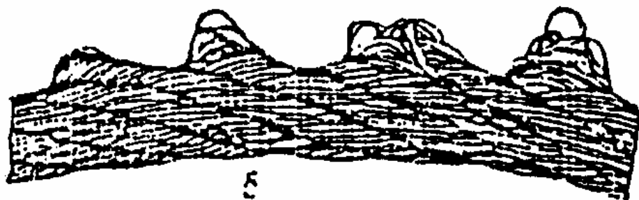
Рис.5. Выдавливание проволок прядей. а – в одной пряди, б – в нескольких прядях
