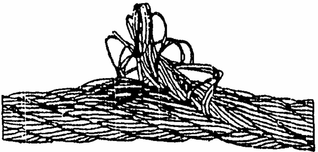
Рис.4 Выдавливание сердечника
